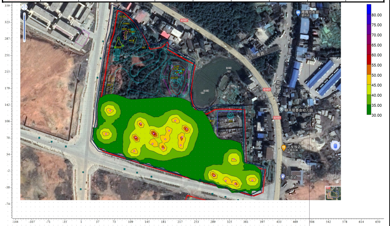
图 4-1 厂界噪声预测等值线图
