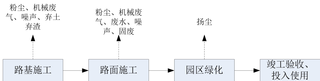
图2-5 道路施工期施工工艺流程及其产污示意图
