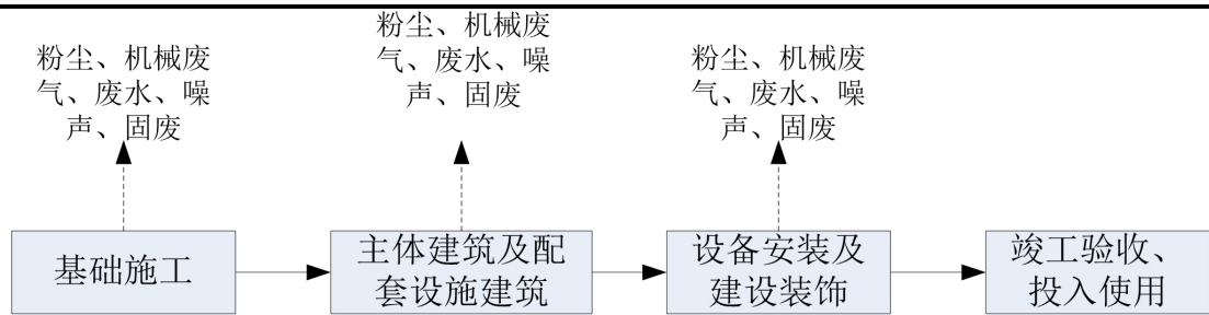
图2-3 地面构筑物施工期施工工艺流程及其产污示意图
